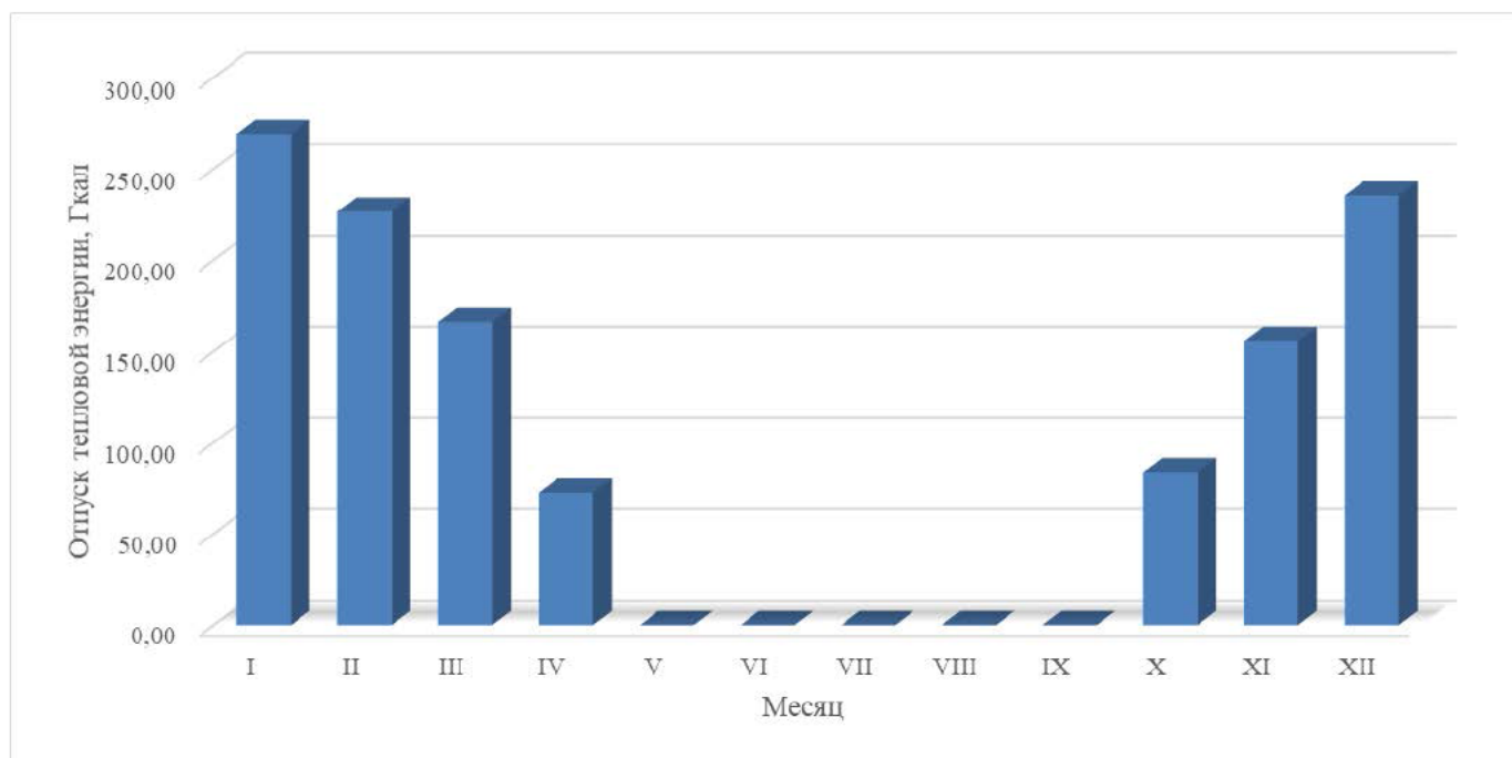
Рисунок 1.4 – Оптимальный температурный график отпуски тепловой энергии для котельной №2
